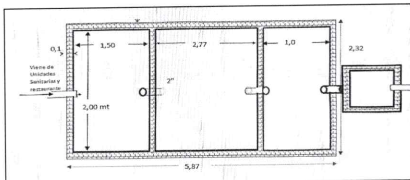
Esquema Tanque Séptico vista en Perfil
