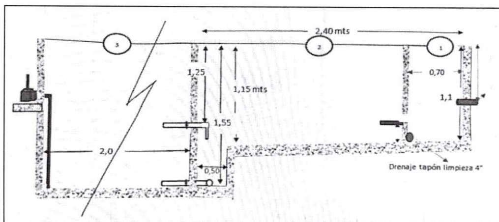
Vista en Perfil del Sistema de Recirculación – Lecho de Secado
