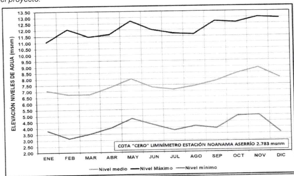
Figura 38. Distribución de los caudales máximos instantáneos mensuales multianuales en el río San Juan, estación hidrológica Noanama Aserrió y transpuestos a los muelles Potedó y Cocové. Período 1966-2015.
