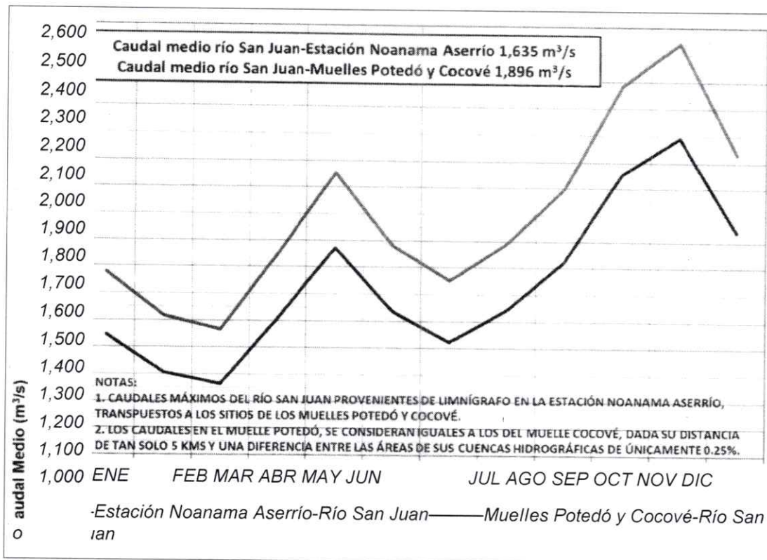
Figura 37. Distribución de los caudales medios mensuales multianuales en el río San Juan, estación hidrológica Noanama Aserrío y muelles Potedó y Cocové. Período 1966-2015. Fuente: IDEAM.
