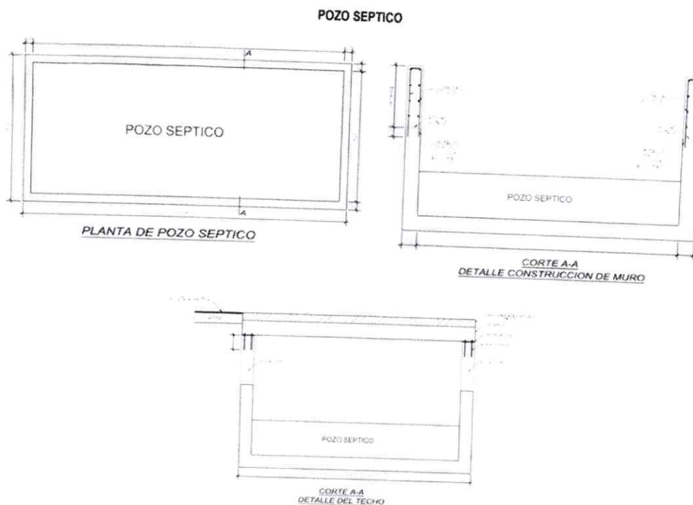
Figura 1 Diseño del tanque séptico Fuente: expediente Finca La Bendición PZ
