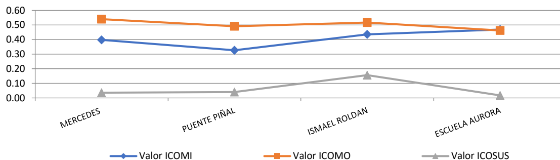
Figura. índices de contaminación Quebrada Aurora época seca.
